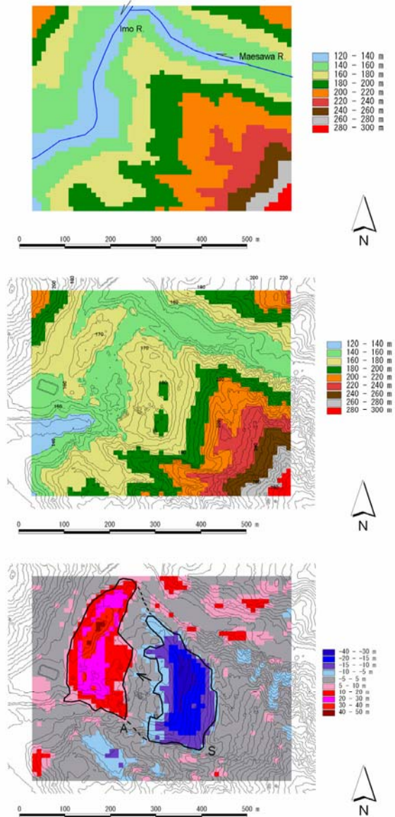
図一六 東竹沢地すべりの標高変化
