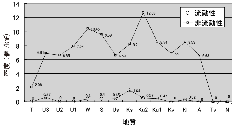
図一五 各地質の斜面崩壊密度
