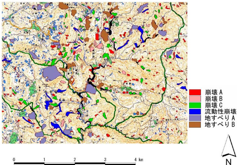
図-2 斜面崩壊6タイプの分布
