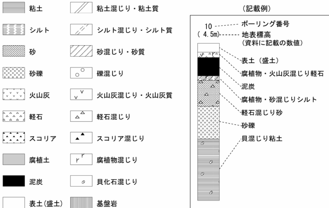
図 - 1 ボーリング柱状図の凡例
