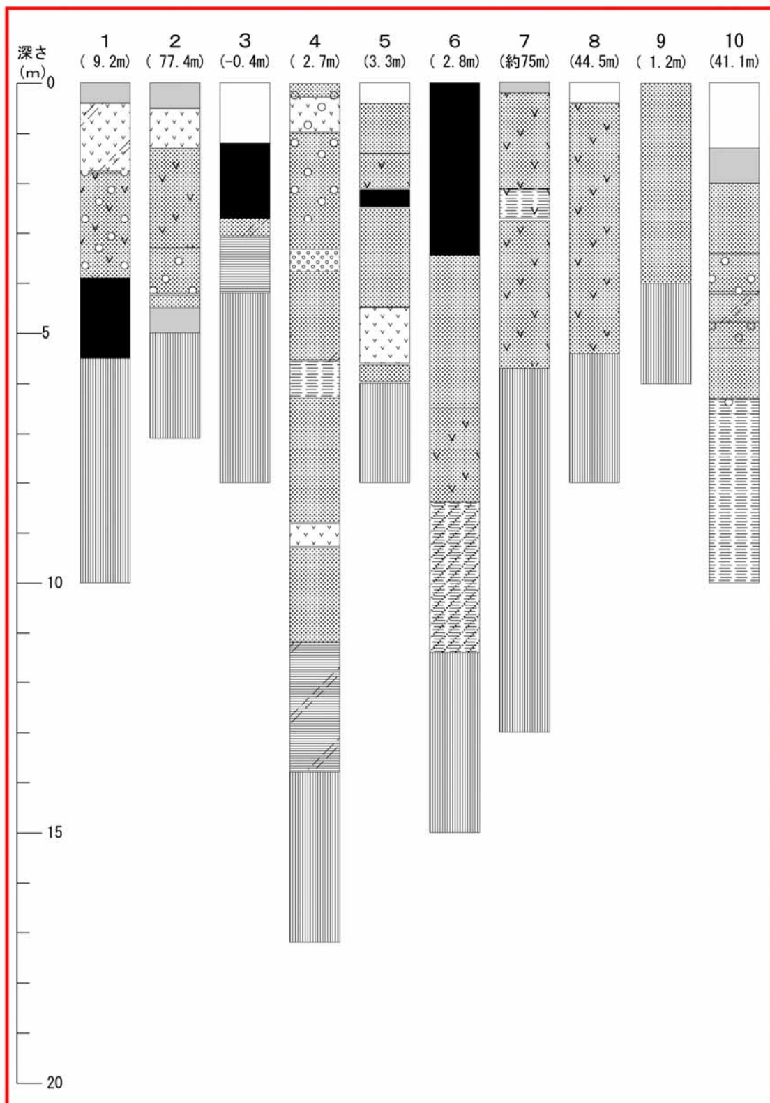
図 - 3 ボーリング柱状図 ( 1 )
