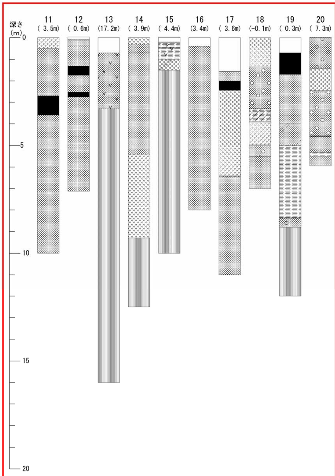
図 - 4 ボーリング柱状図 ( 2 )
