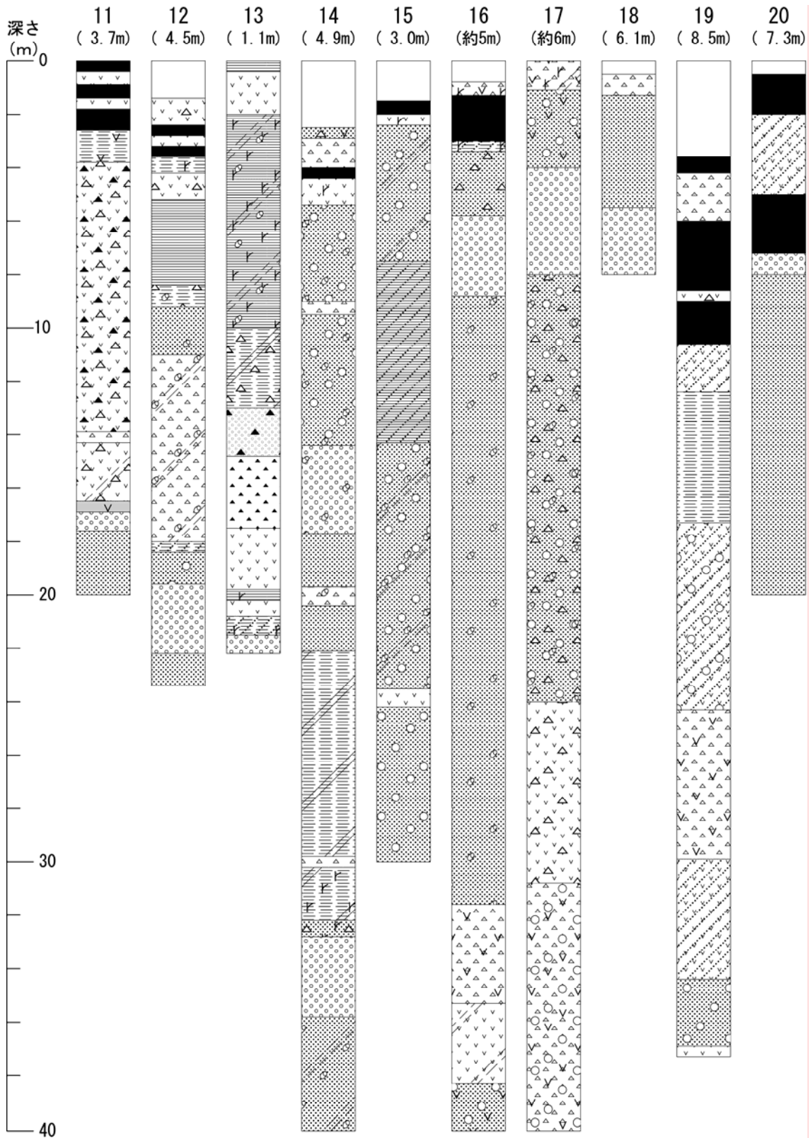
図 29 ボーリング柱状図 (2) (No. 16、17 のボーリング地点の標高は、1 : 5000 「苫小牧都市計画図」 (苫小牧市) による)
