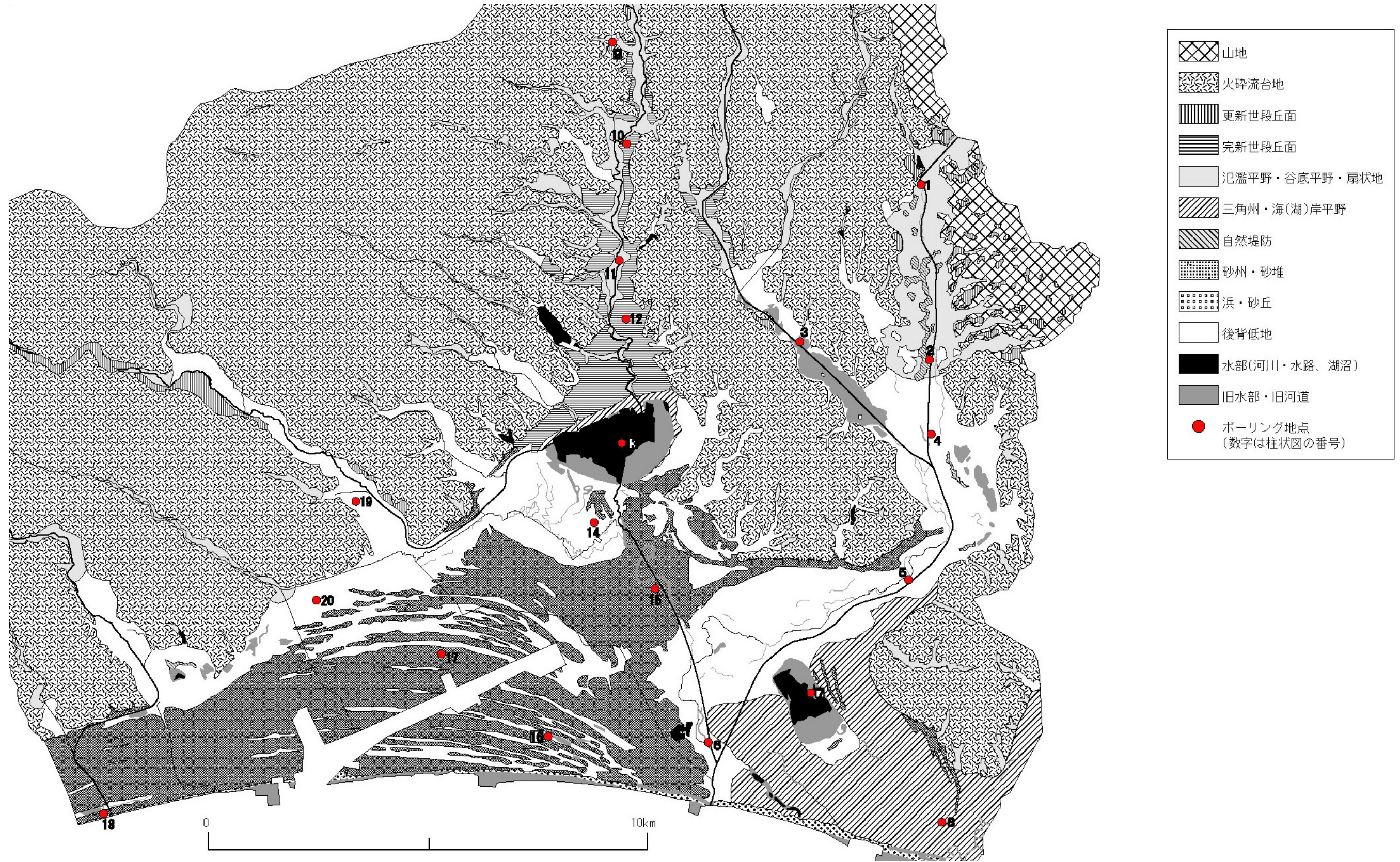
図 27 ボーリング位置
