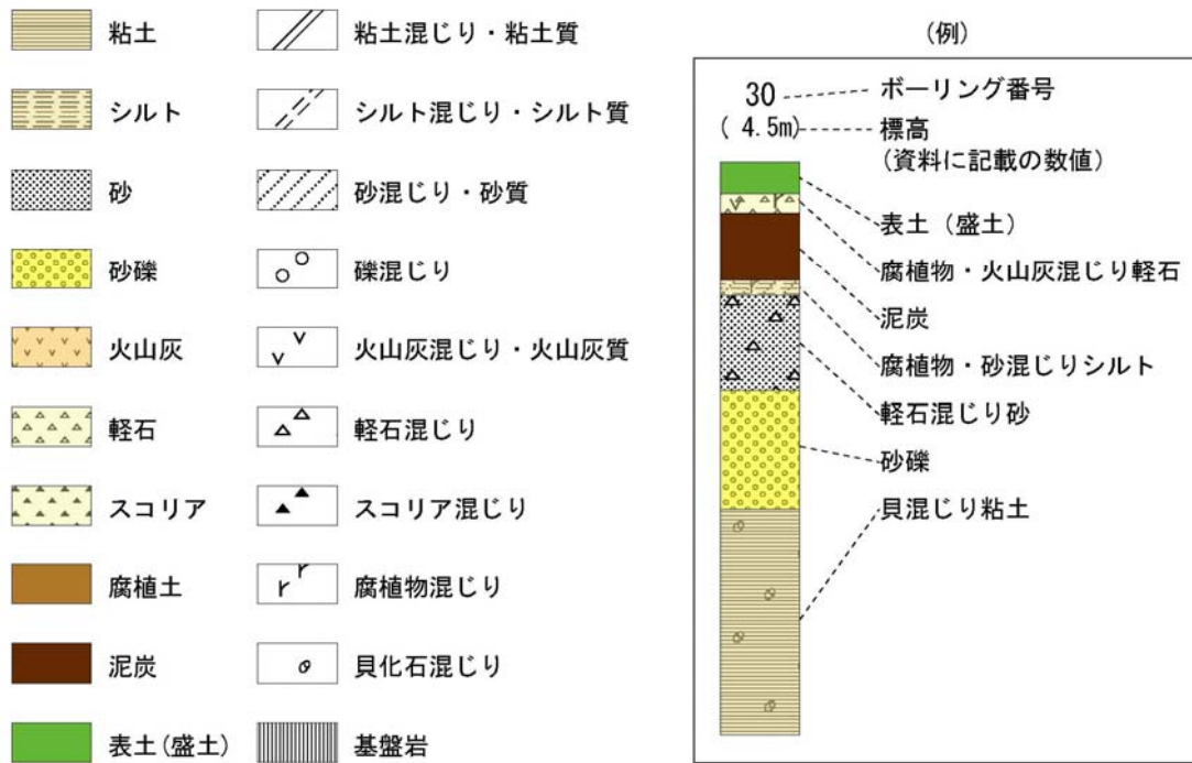
図 26 ボーリング柱状図の凡例
