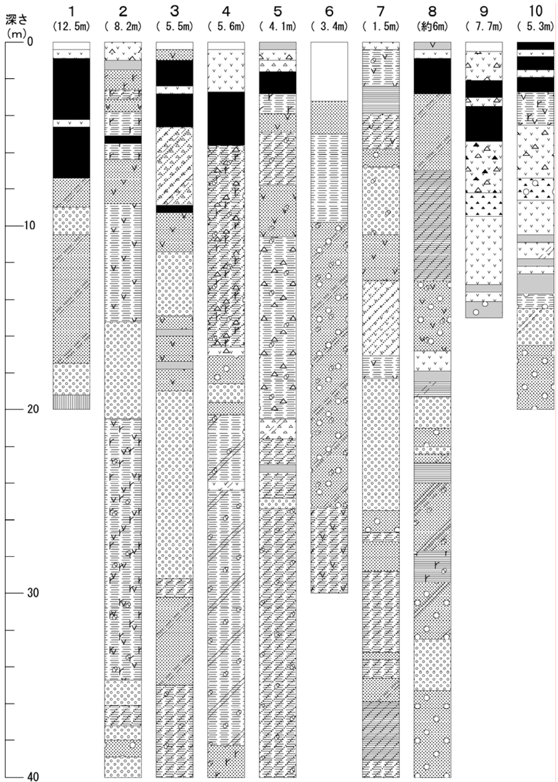
図 28 ボーリング柱状図 (1) (No. 8 のボーリング地点の標高は、1 : 2500 「苫小牧東部地域地形図」 (株式会社苫東) による)
