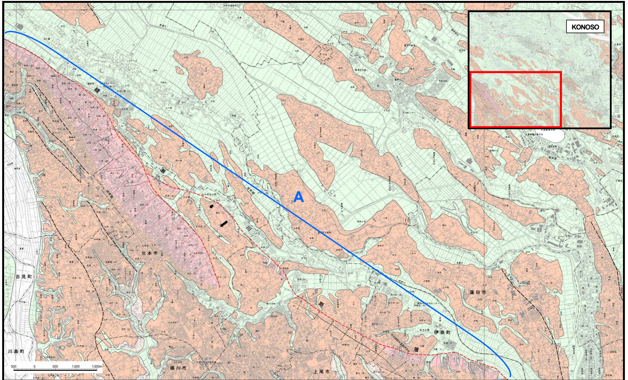
A: Ayasegawa Fault
