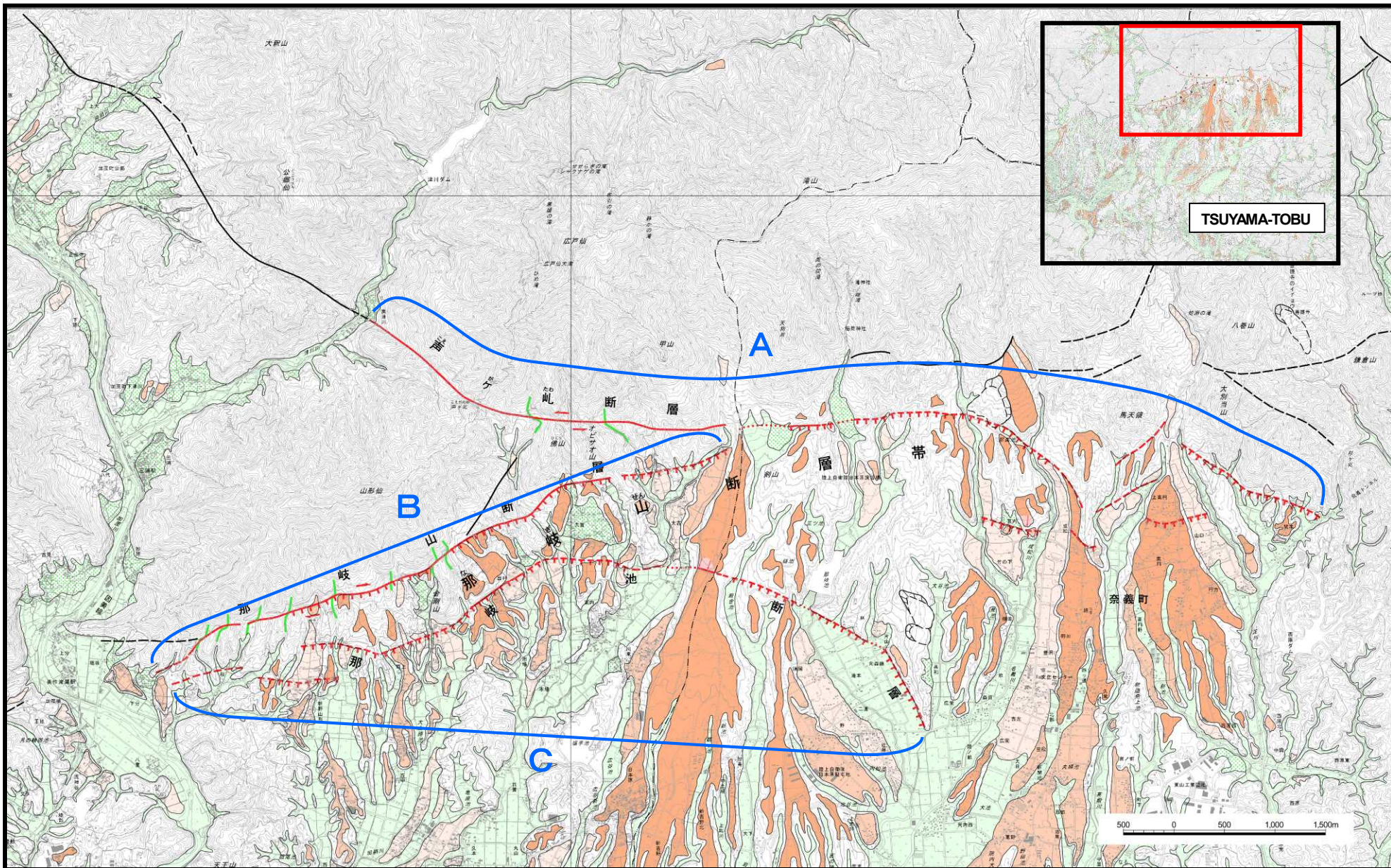
A: Koegatawa Fault
