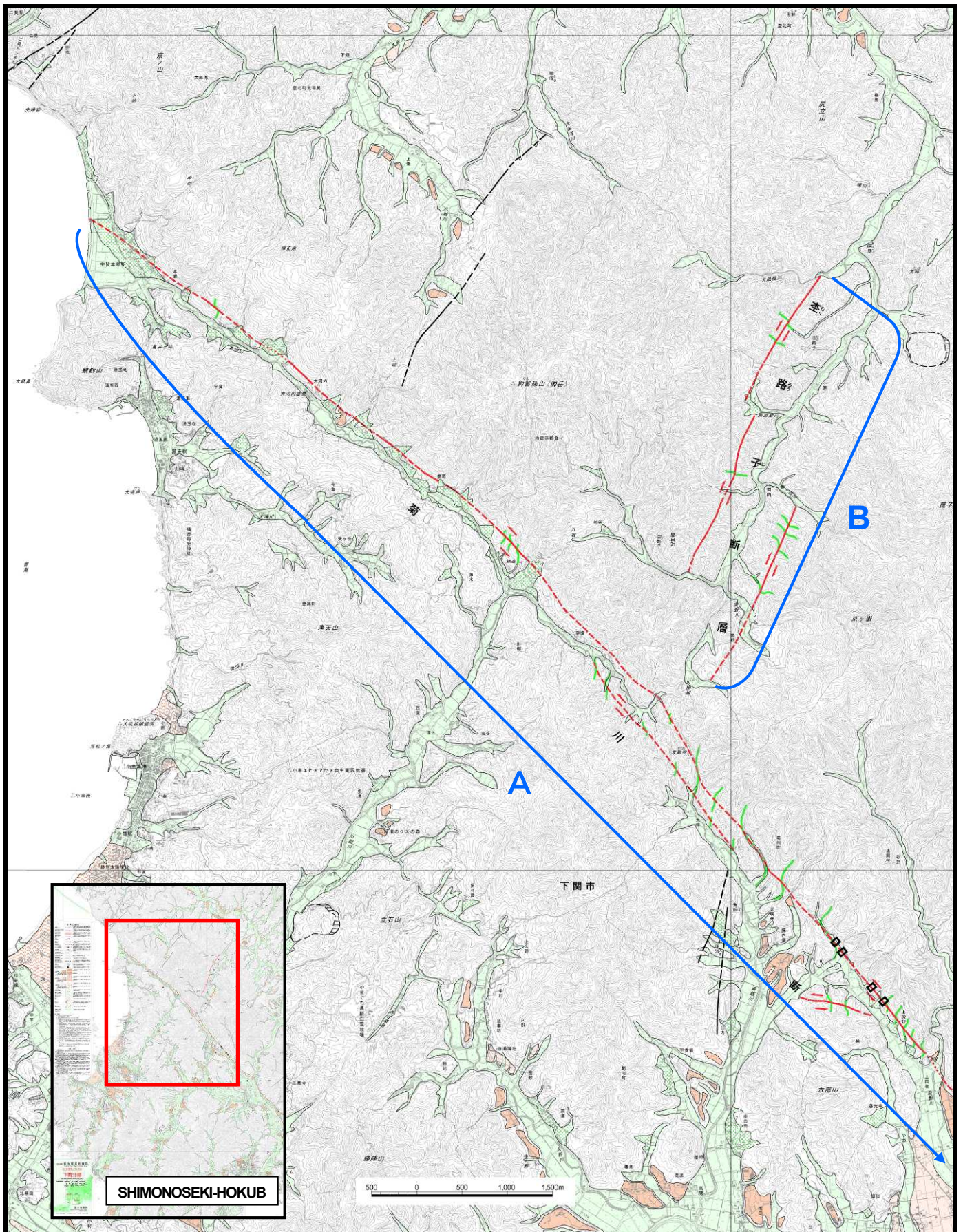
A: Kikugawa Fault B: Mukuroji Fault
