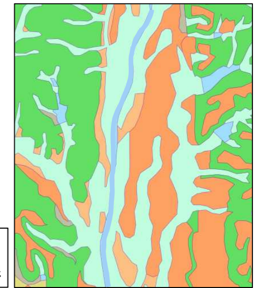
図2 地形分類図 (2万5千分1土地条件図)
