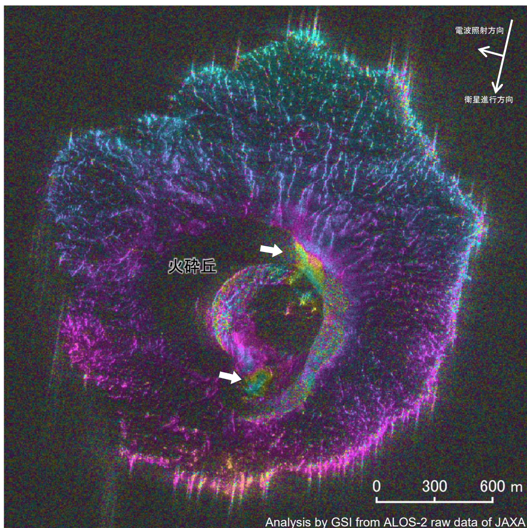
図1 SAR干渉解析結果
